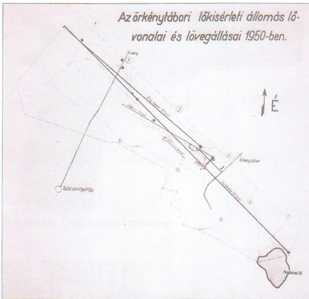
8. számú kép. Az örkénytábori lökisérleti állomás lövonalai és lövegállásai 1950-ben
