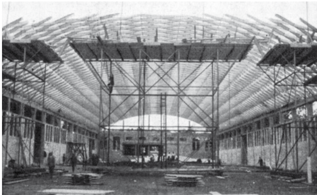
A nagy lovarda tetőszerkezetének összeszerelése (Tér és Forma, 1931. április)
